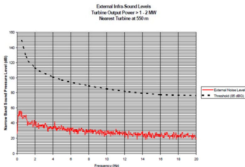
Фиг. 19-в. Спектр на излъчвания инфразвук от вятърни турбини с мощност 1-2 MW, измерен на разстояние 550 м от турбината
