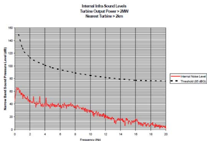
Фиг. 19-б. Спектър на излъчвания инфразвук от вятърни турбини с мощност >2 MW, измерен на разстояние 2000 м от най-близката турбина
