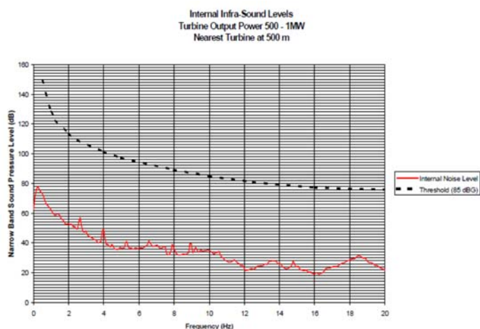
Фиг. 19-а. Спектър на излъчвания инфразвук от вятърни турбини с мощност 500 kW ÷ 1 MW, измерен на разстояние 500 м от тях
