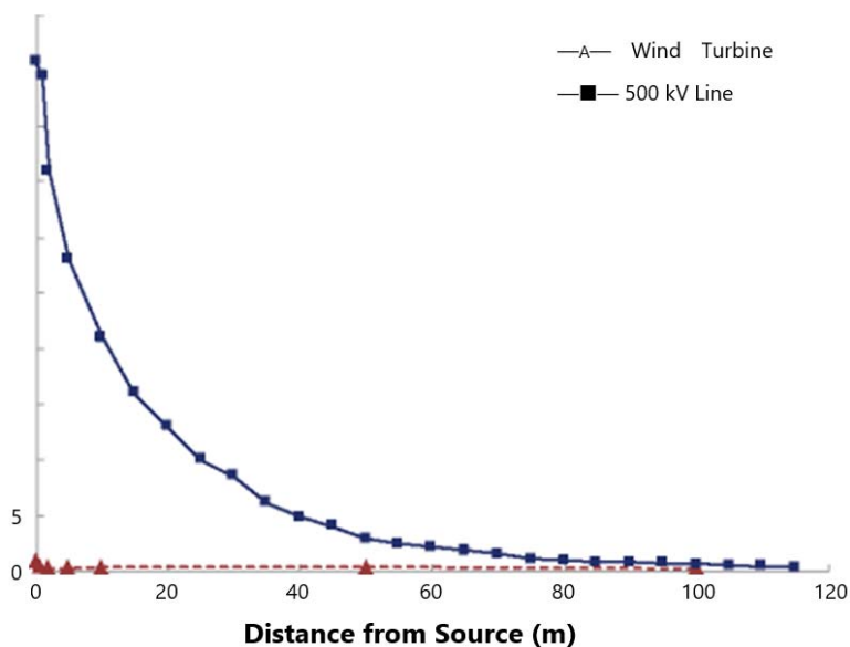
Фиг. 3. Сравнение между магнитните полета, измерени до турбините и полетата, измерени до въздушен електропровод 500 kV
