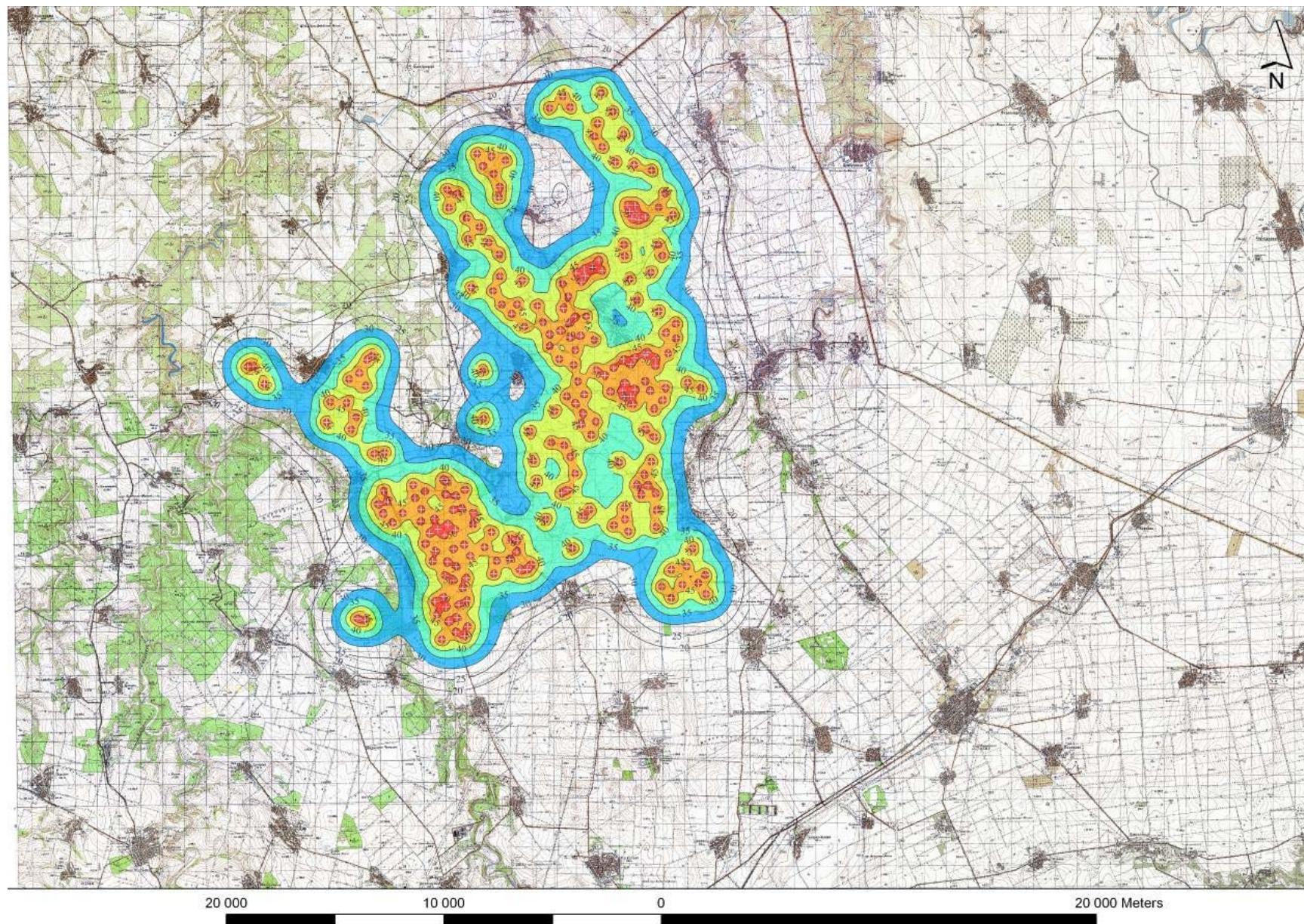
Фиг. 10. Шумова карта на територията, предвидена за изграждане на ВятрЕЦ "Крушари" и на останалите паркове, включени в кумулативната оценка. Картата отразява шума, генериран от едновременната работа на 229 вятърни турбини и 3 подстанции.
